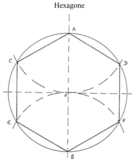
Fig. 1, Hexagone régulier inscrit. Fig.2, Sceau de Salomon.
